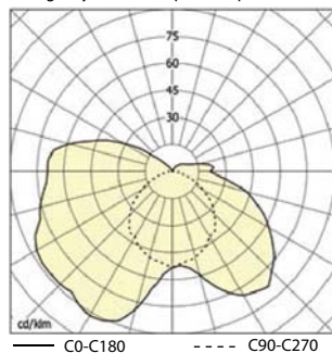
VIPET-N-Em, 2x36W, IP 66 Emergency mode/ Аварийный режим
