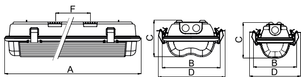
F – spacing of self-locking fastening springs Шаг на крепление самокрепящихся клипсов
